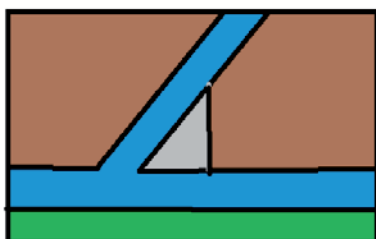
Een Hörntje: een punt van het perceel wordt afgegraven met een flauw talud
