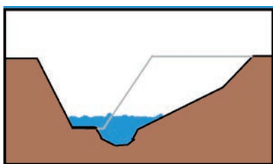
Dwarsdoorsnede: meer ruimte voor vis-sen, amfibieën en meer waterbergingsruimte
